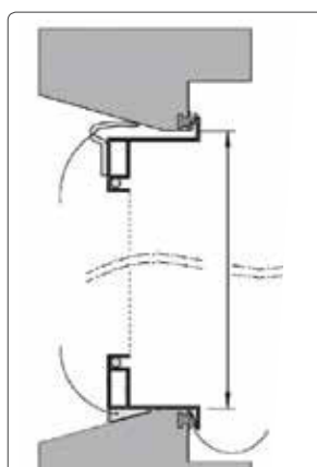
Type C Plastvindue -m/ knækket int. sålbænk
