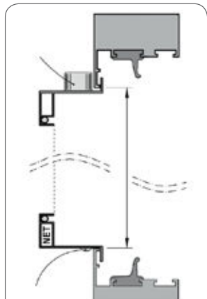
Type ALU Aluvindue -tynd karm kant
