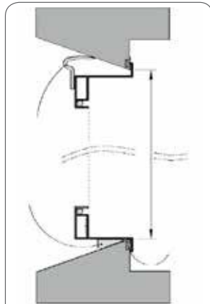
Type B Plastvindue -m/ lige int. sål- bænk
